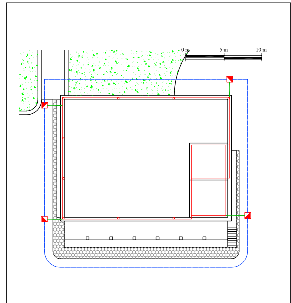
SCHEMA IMPIANTO ANTIFULMINE RESIDENZA DELL'AMBASCIATORE
