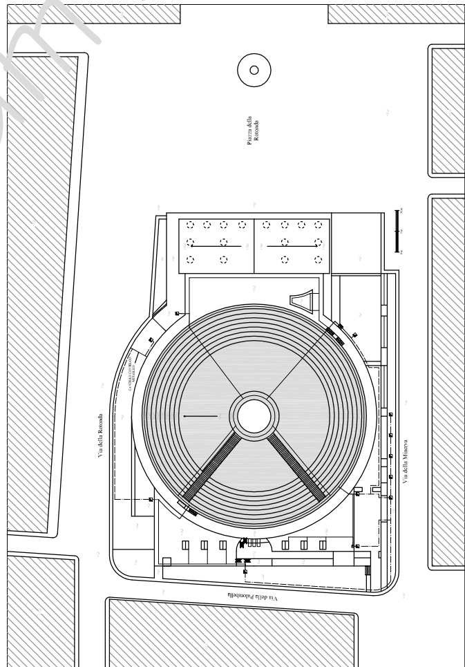
SCHEMA IMPIANTO ANTIFULMINE PANTHEON
